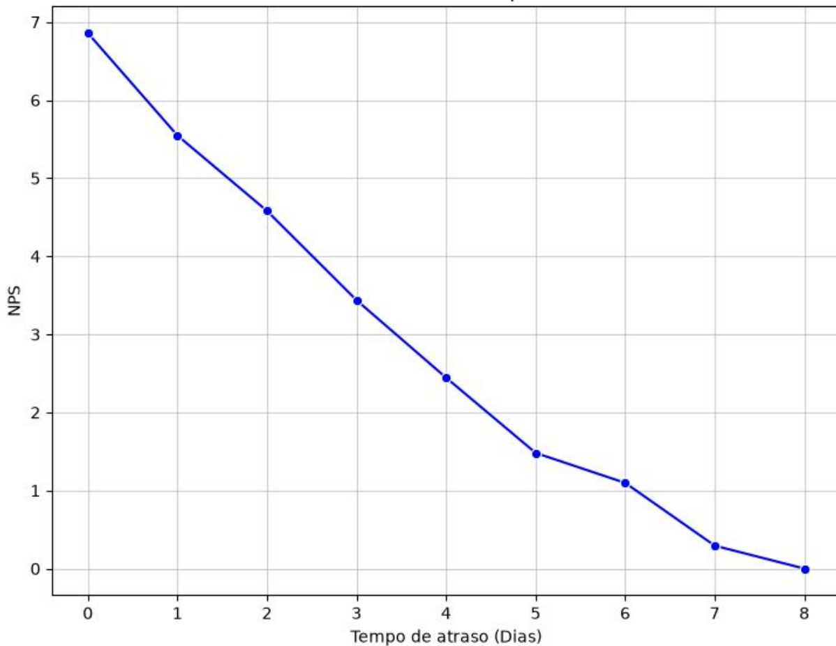
Nota Média do NPS x Tempo de Atraso
